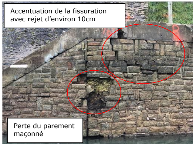
Décollement et perte du parement avec fissures et rejet - Photos 2019 et 2020
