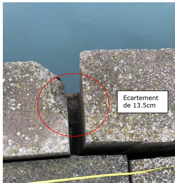
Fissure au niveau de la longrine- Photos 2019 et 2020
